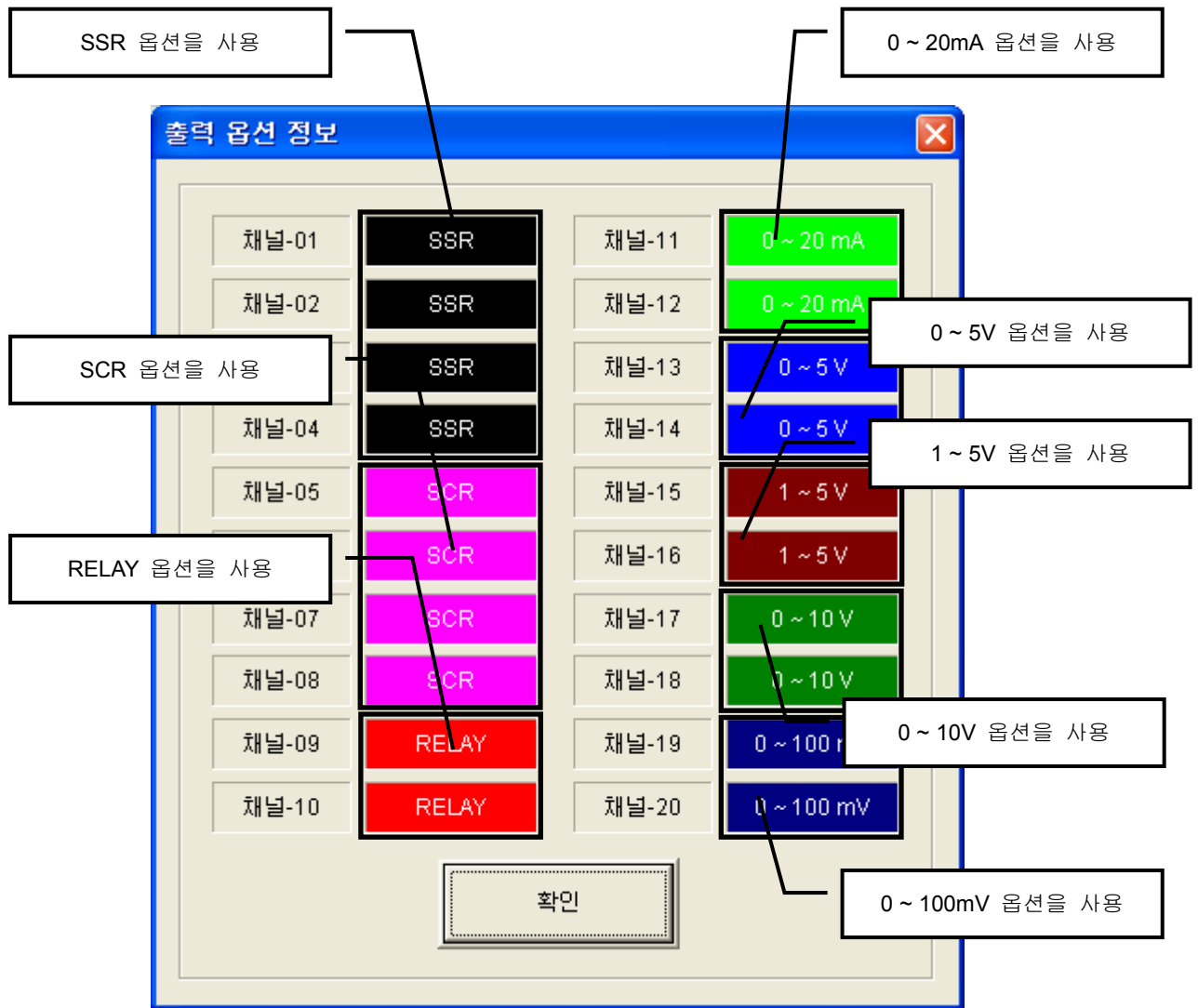
(그림 4) 출력 옵션 정보 화면
