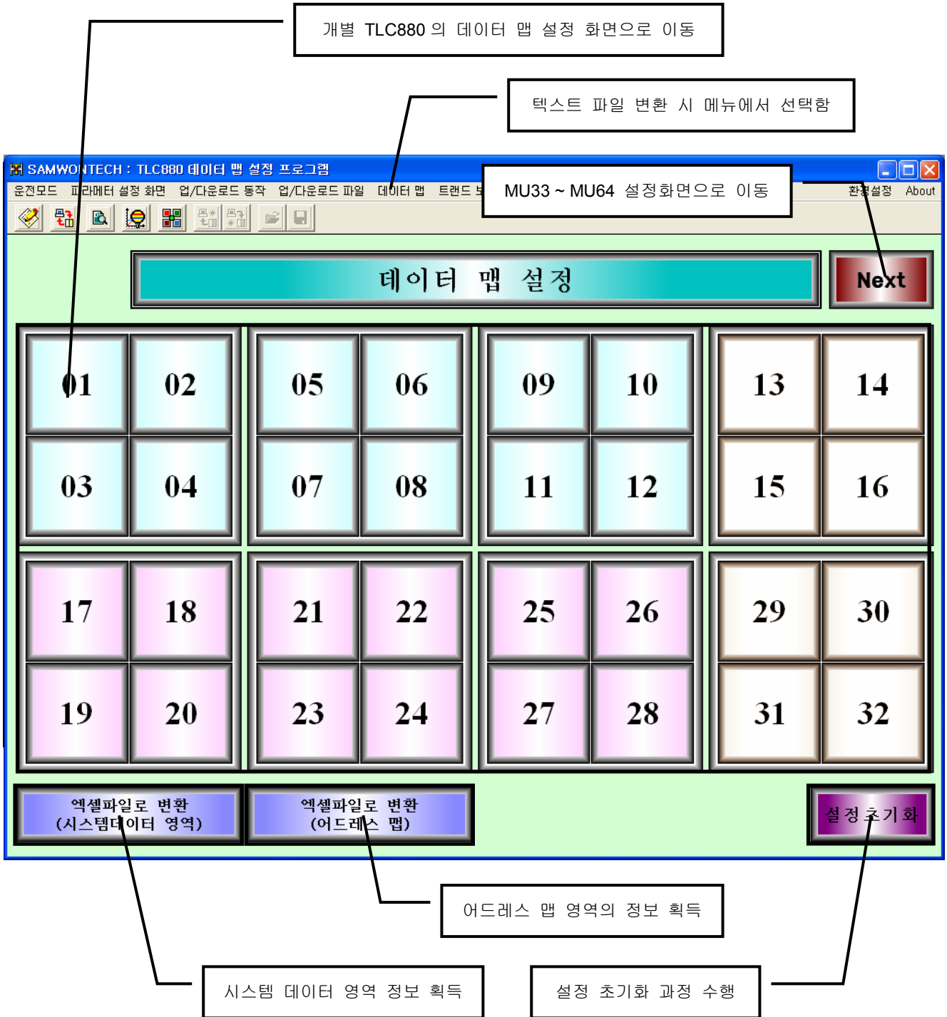
(그림 38) 데이터 맵 설정 화면 구성
